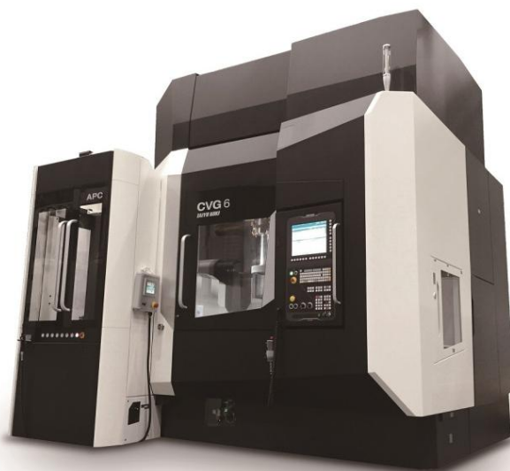
CNC立形複合研削盤 CVG-6
